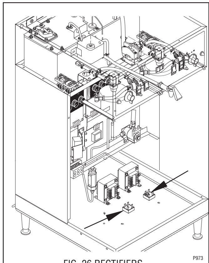
FIG. 26 RECTIFIERS P973
